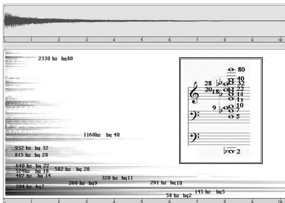
EXEMPLE 7. Sonagramme du sib grave d'un piano à queue
