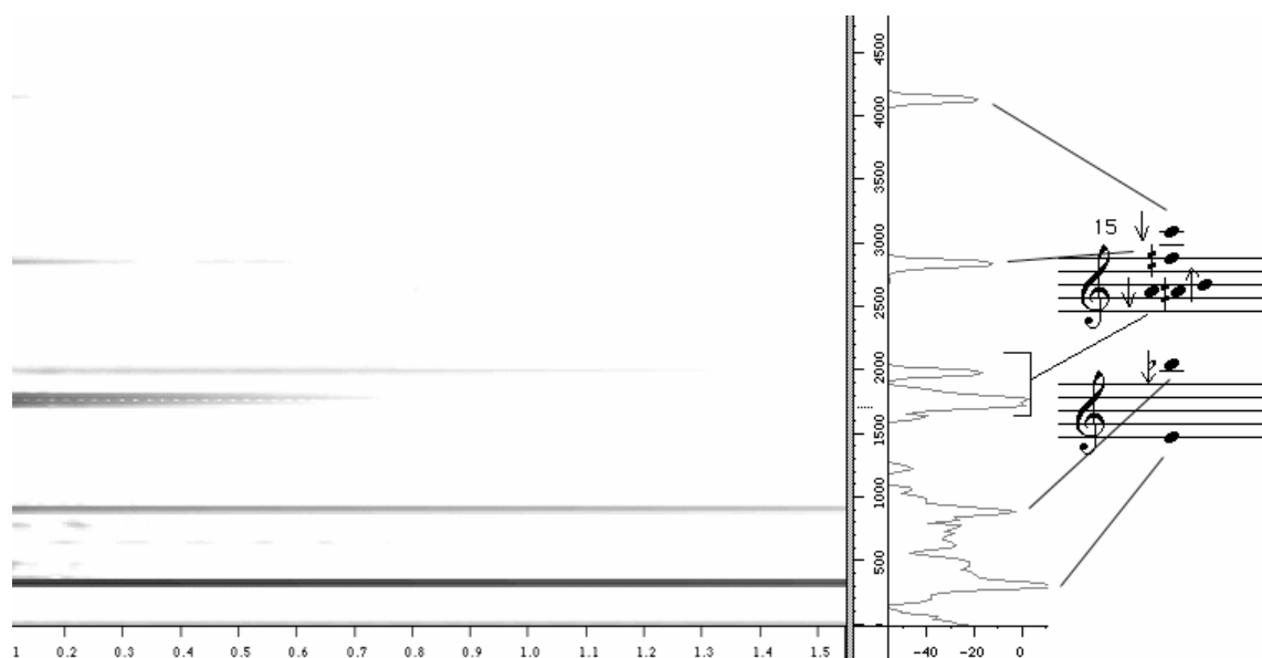
EXEMPLE 9. Spectre de bonang et sa transcription en hauteurs microtonales
